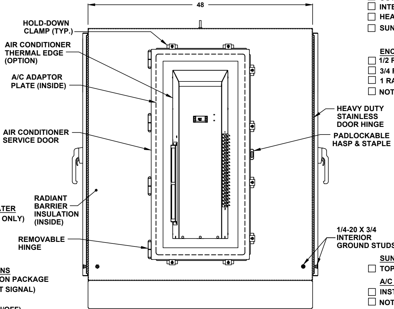
LEFT SIDE
